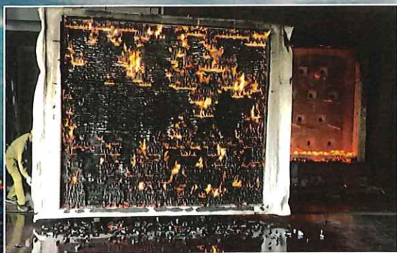
▲防耐火試験
