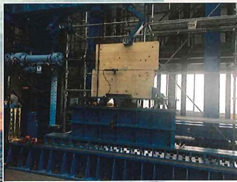
▲構造強度試験
