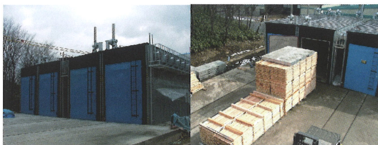
高温蒸気乾燥機 4基 乾燥容量 32 m 3 最高温度 120℃
